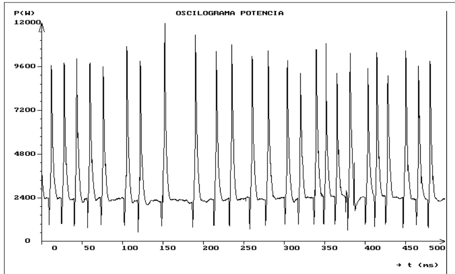
Fig. 8 - Oscilograma de Potência
