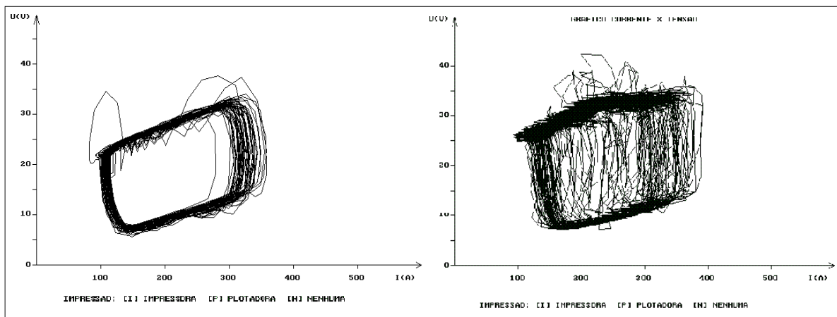
Fig. 12 - Gráfico Tensão X Corrente
