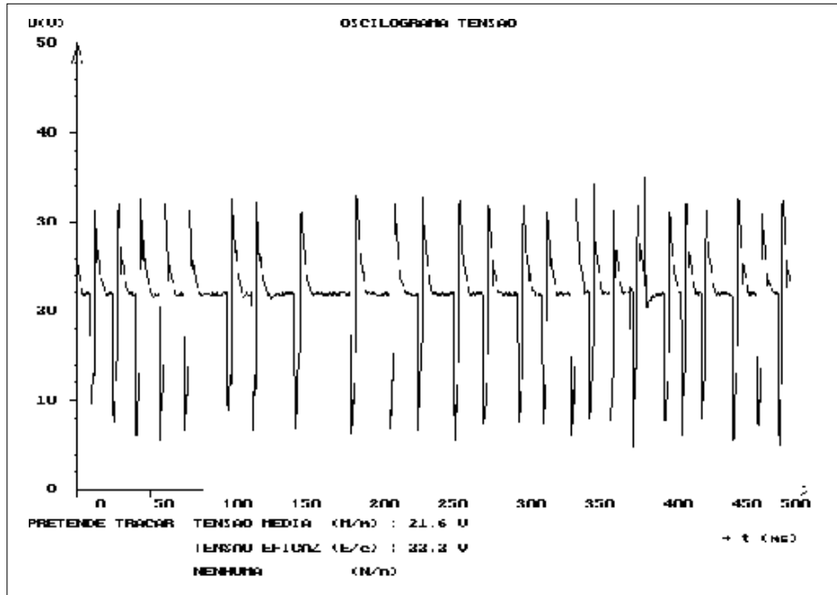
Fig. 7 - Oscilograma de Tensão
